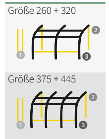
Gestängeskizze - Serienausstattung - empfohlene Zusatzausstattung
